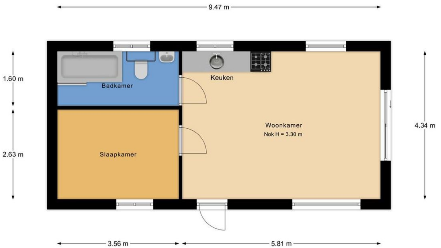
Bijgebouw Begane grond
